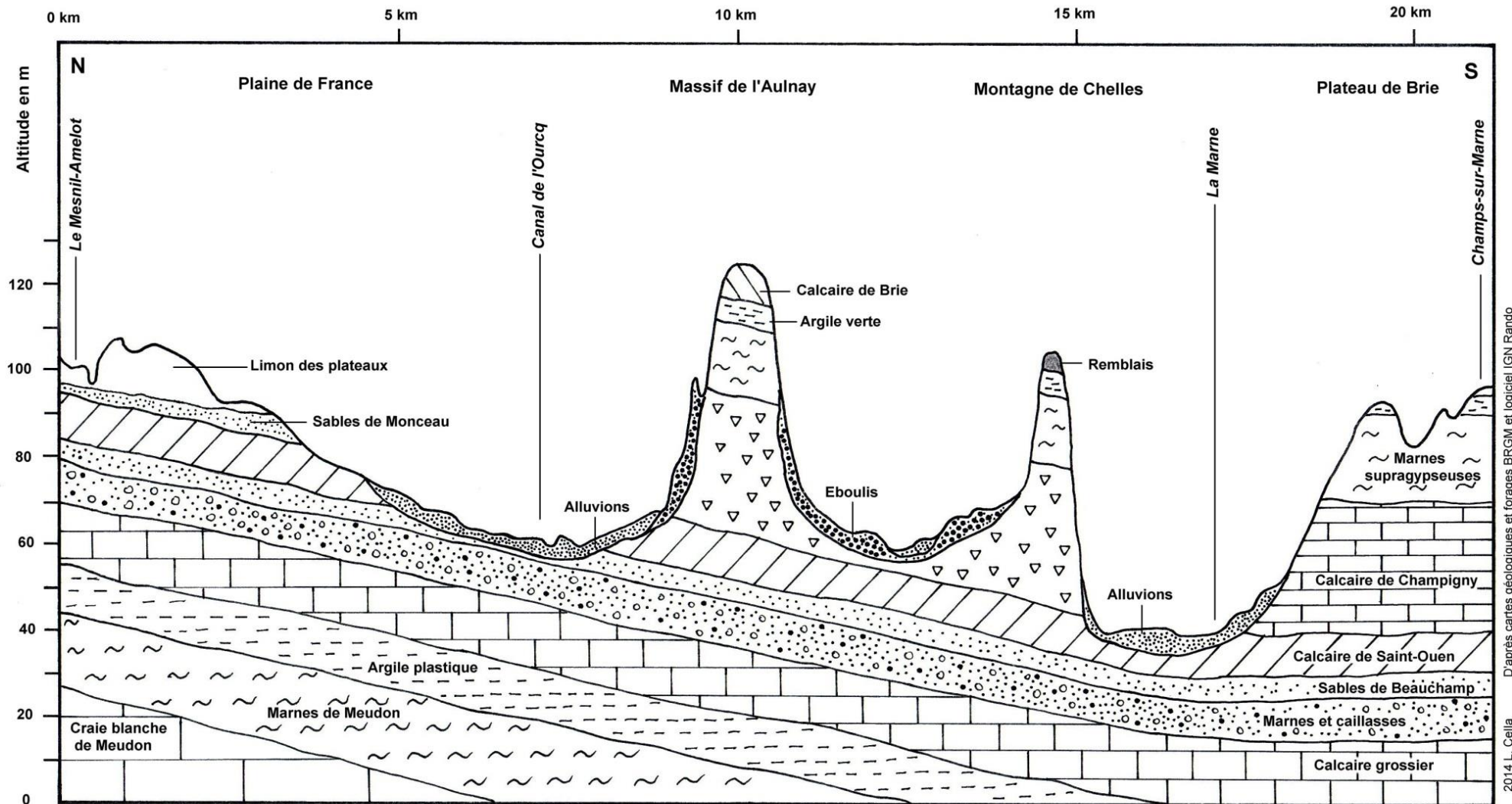
Figure 2 : Coupe Nord-Sud de la zone de Chelles
