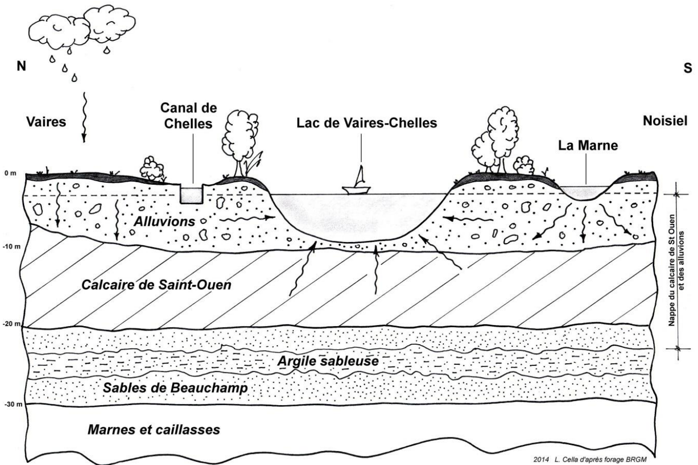
Figure 3 : Alimentation du lac de Vaires-Chelles par la nappe phréatique.
