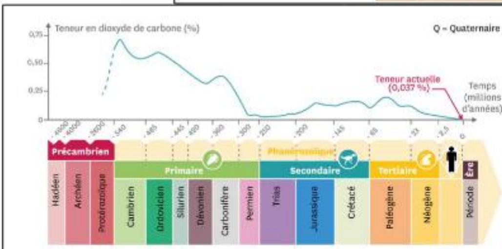
Document 11 : Les variations de la concentration dioxyde de carbone CO2 atmosphérique au cours des temps géologiques
